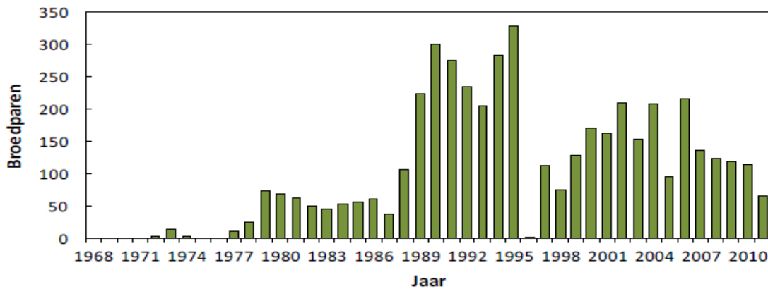
Figuur 19: Aantal broedparen van de Lepelaar in de Oostvaardersplassen in de periode 1968-2011. Uit Beemster et al. 2012 met als databron Waterdienst RWS.
