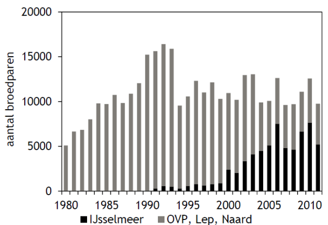
Figuur 22: Aantalsontwikkeling van de Aalscholver kolonies in het IJsselmeer en van kolonies rondom het Markermeer die van het IJsselmeer afhankelijk zijn (Oostvaardersplassen, Lepelaarplassen en Naardermeer), uit Boele et al. 2013.
